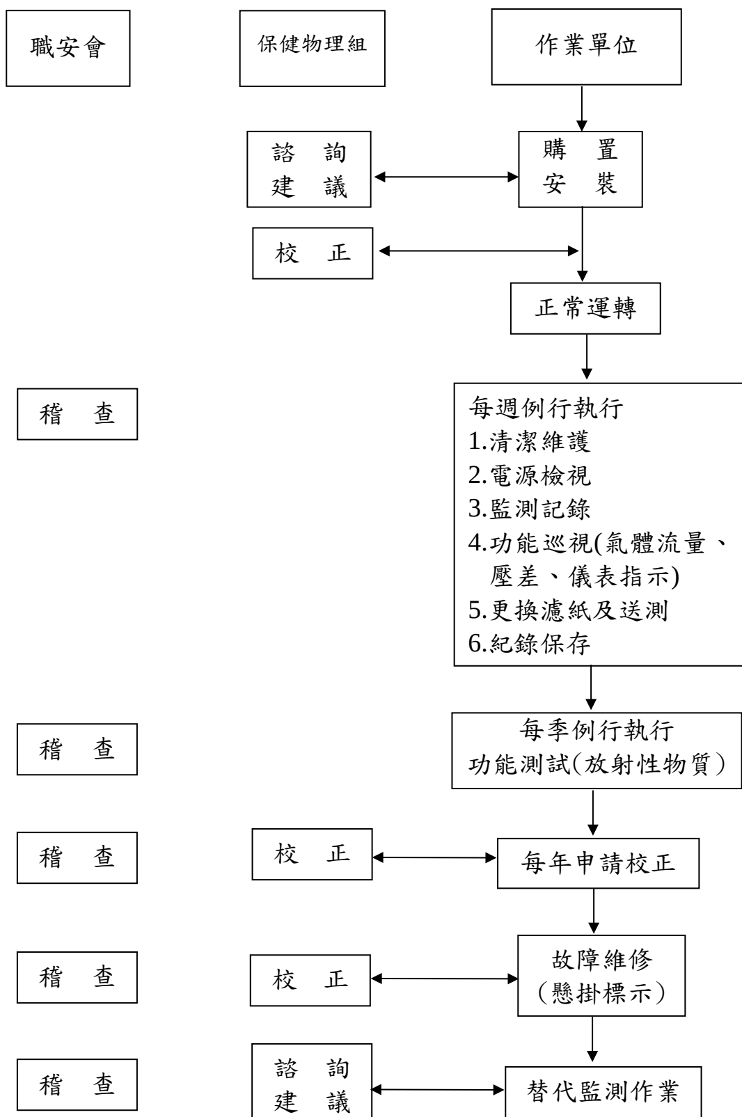
圖 7.1 核能研究所輻射作業區輻安監測儀器例行檢查功能測試、校正、稽查作業分工圖
